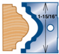
#4545 Astragal
